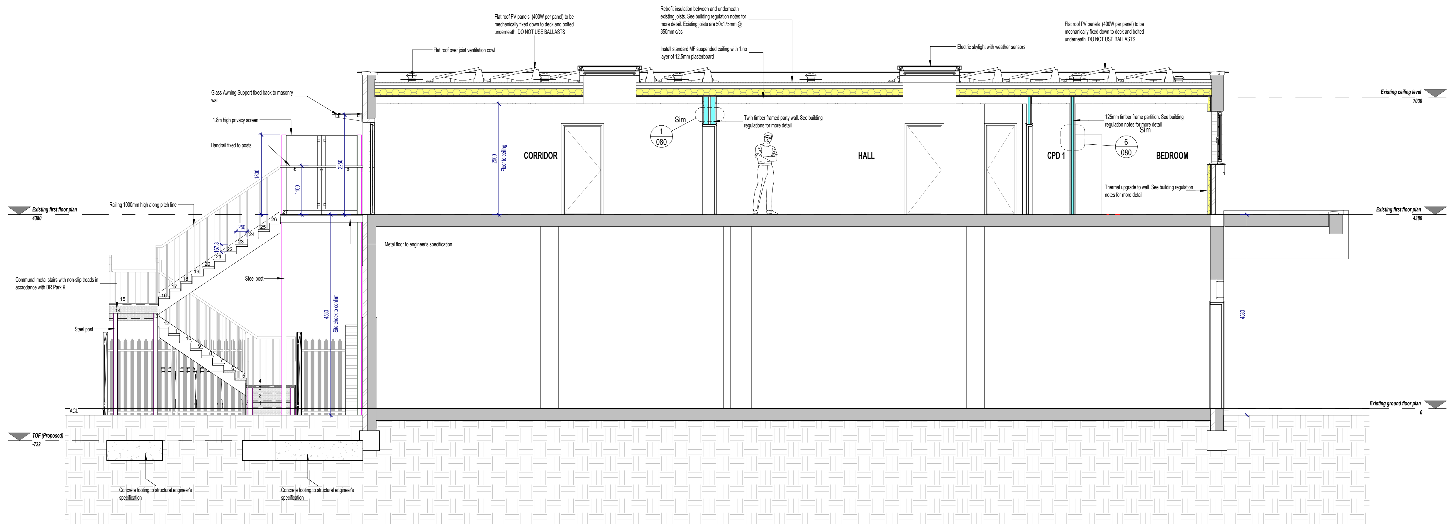
1 Section A-A 1:50
