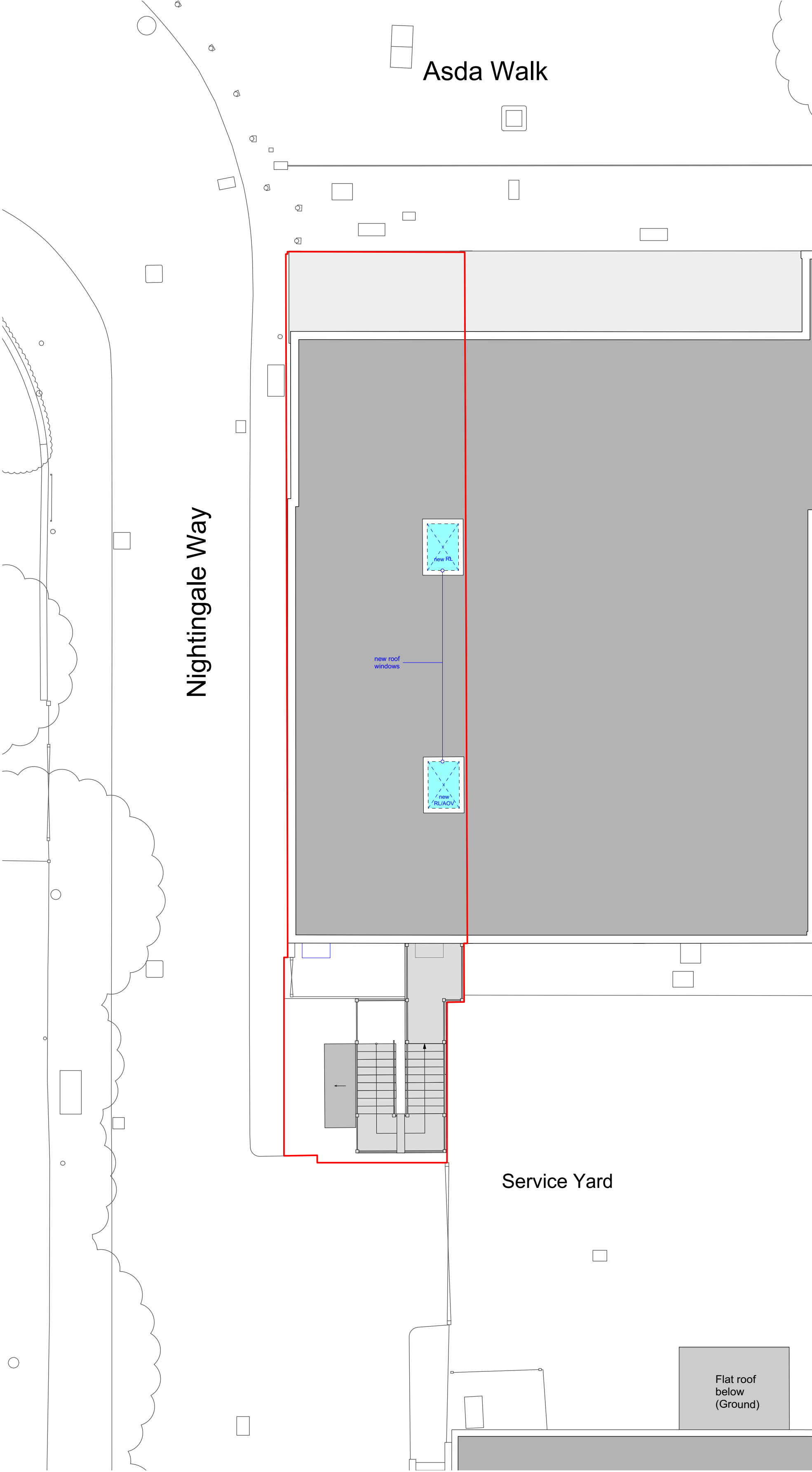
5 Roof Scale: 1:100
